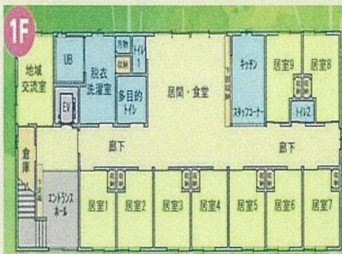
グループホーム平面図の一例
